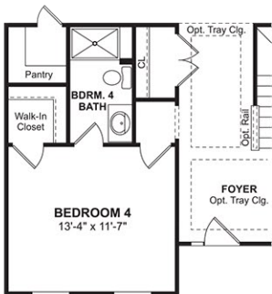
OPTIONAL BEDROOM 4/BATH 4
